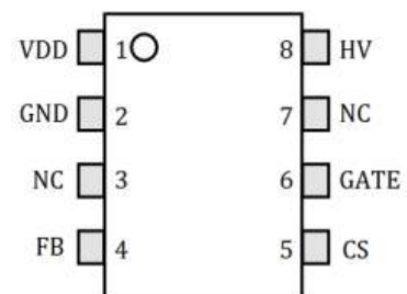
SOP-8俯视图
